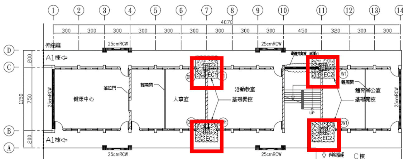
B 棟 1FL 補強位置平面圖
